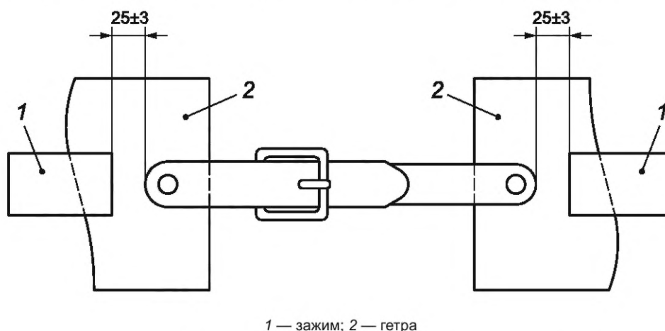
Рисунок 2 — Пример для испытания на прочность систем застежек
